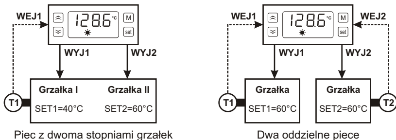
Piec z dwoma stopniami grzałek
