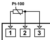
czujnik Pt-100 3-przewodowy
