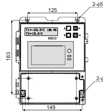
Rys.2 Wymiary obudowy rejestratora.
