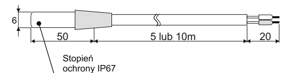
Rys.4. Wymiary czujnika przewodowego.
