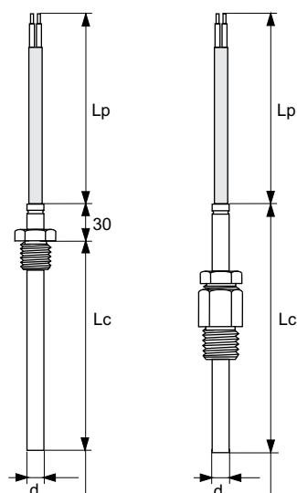
z króćcem stałym
