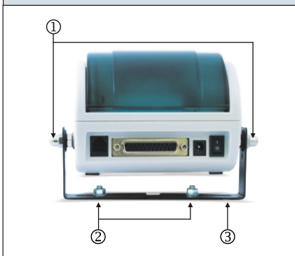
Rys.2 Uchwyt montażowy (3).
